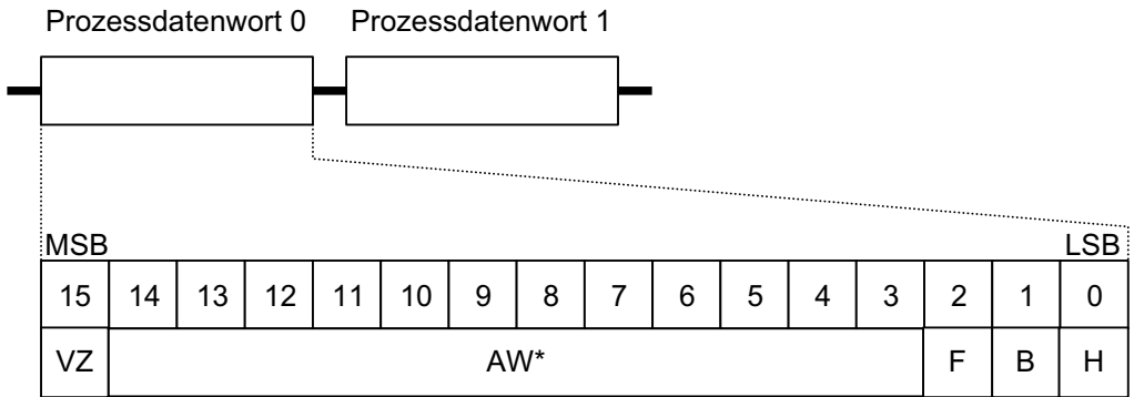
Bild 8 Prozessdaten-Eingangsworte
