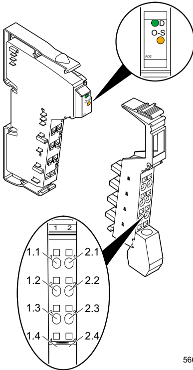
Bild 2 VARIO AO 2/U/BP mit zugehörigem Stecker
