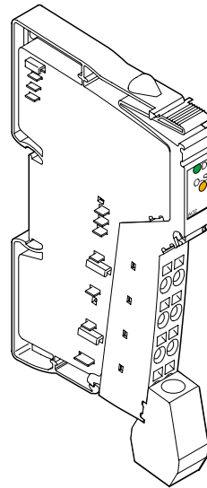
Bild 1 Das Modul VARIO AO 2/U/BP mit aufgesetztem Stecker
