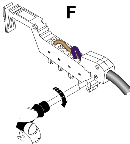
Bild 6 Anschließen des Schirmes über den Schirmstecker
