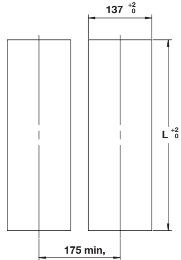
Übereinandermontage (vertikal, max. 3 Einheiten)
