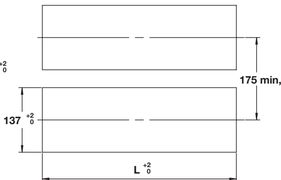
Nebeneinandermontage (horizontal)
